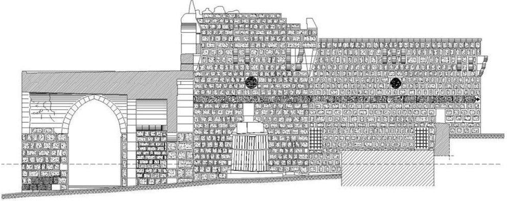
Çizim 2. 1-1 Kesiti
