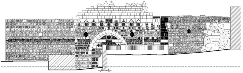
Çizim 4. Doğu Cephesi
