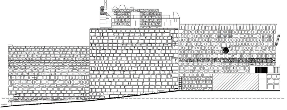
Çizim 6. Güney Cephesi
