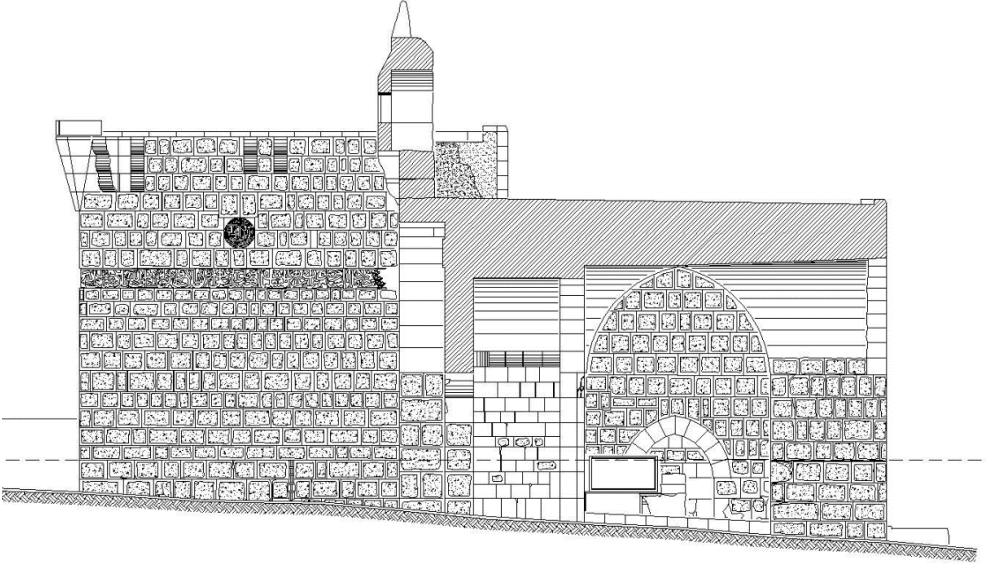
Çizim 3. 2-2 Kesiti
