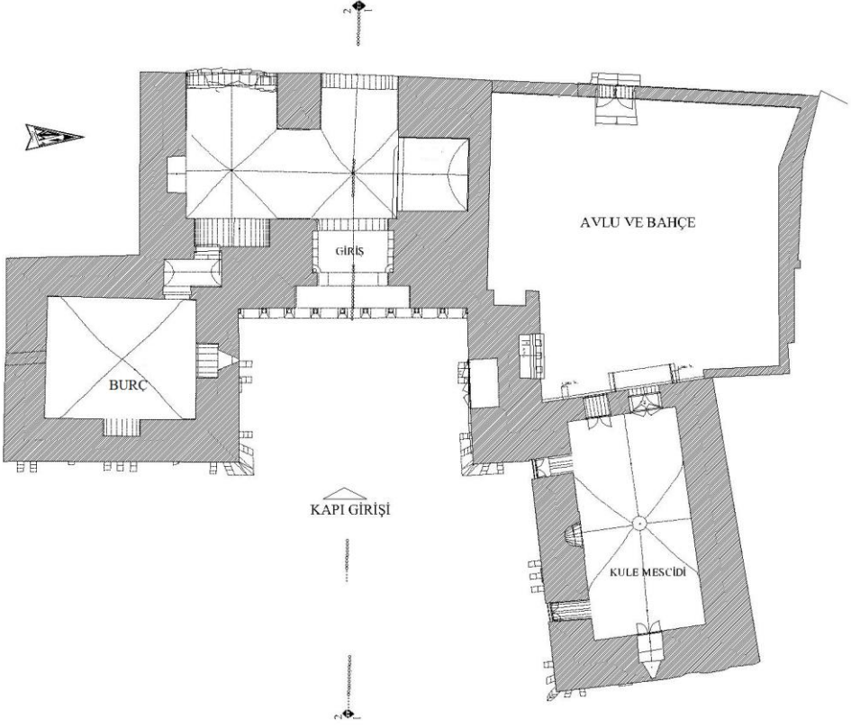
Çizim 1. Urfa Kapısı –Plan (Şanlıurfa Vakıflar Bölge Müdürlüğü arşivinden 11 )
