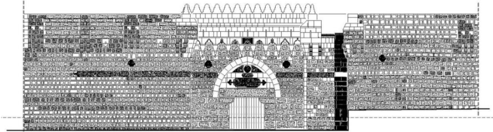
Çizim 16. Doğu Cephesi – Restitüsyon
