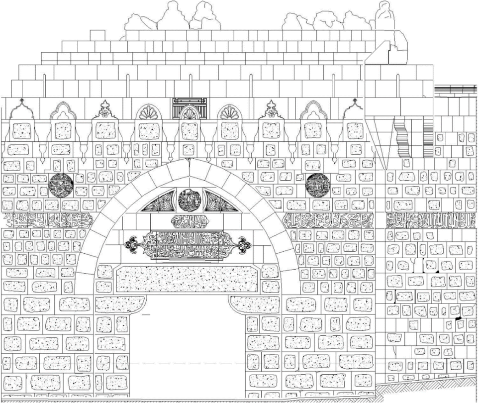
Çizim 7. Doğu Cephesi-Giriş Kapısı-Detay
