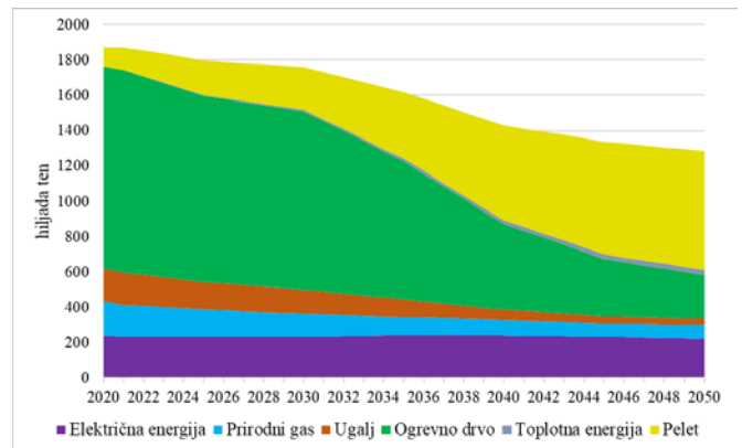
Slika 9. Finalna potrošnja za Scenario 2 – kombinacija svih instrumenata
