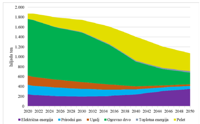
Slika 10. Finalna potrošnja za Scenario 3 – kombinacija svih instrumenata [19]
