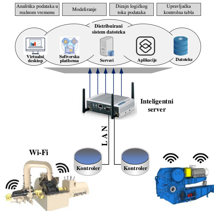
Slika 4. Arhitektura PdM 4.0
