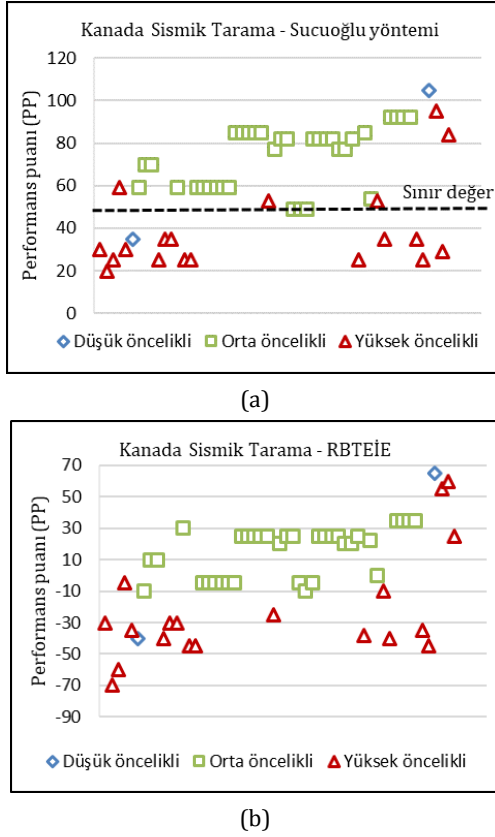
Şekil 3. Kanada Sismik Tarama yöntemine göre hasar riski değişiminin, (a): Sucuoğlu yöntemi, (b): RBTEİE' de önerilen yöntemle karşılaştırılması.
