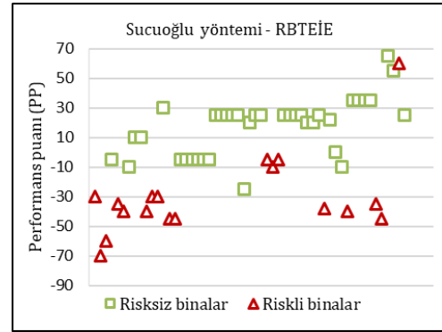
Şekil 4. Sucuoğlu yöntemine göre riskli ve risksiz bina sınıflarının RBTEİE'deki performans puanı değişimleri.
