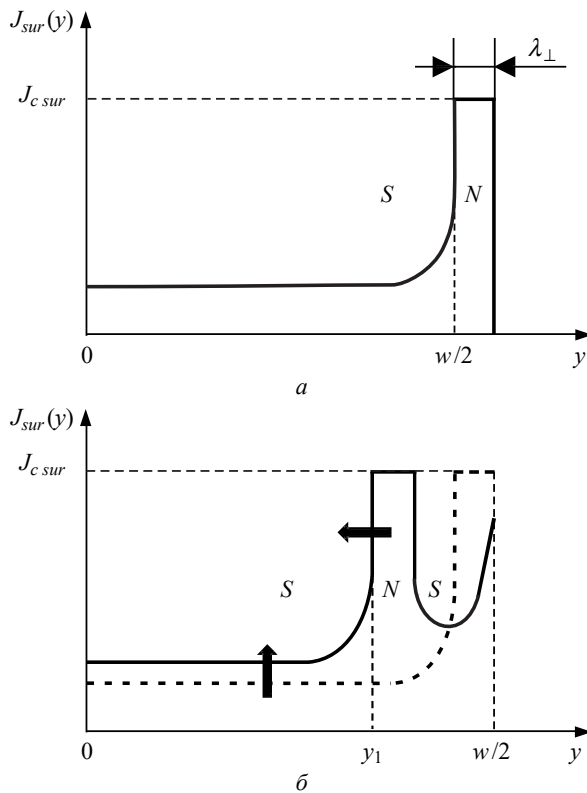
Рис. 3. Еволюція розподілу струму J_{sur}(y) залежно від поперечної координати для випадку «повільного» переміщення S - N -межі y_1 до центру смужки \tau_{des}^{(dc)} > 3\tau_E : a – розподіл J_{sur}(y) в момент вмикання струму ( t = 0 ); b – розподіл J_{sur}(y) в момент часу t < \tau_{des}^{(dc)}
