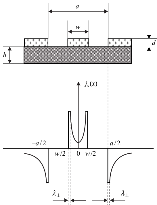
Рис. 4. Розподіл мікрохвильового струму в копланарному хвильоводі: a – ширина хвильоводу; w – ширина центральної смужки; d – товщина надпровідної плівки; h – товщина підкладки
