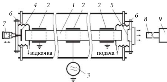
Рис. 2. Схема лазерної установки
