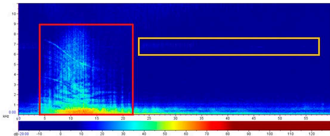
Figura 18. Paisagem acústica da Restinga do Foguete às 16:15h do dia 23/09/2018, indicando biofonia (inseto) em amarelo e antropofonia (avião), em vermelho
