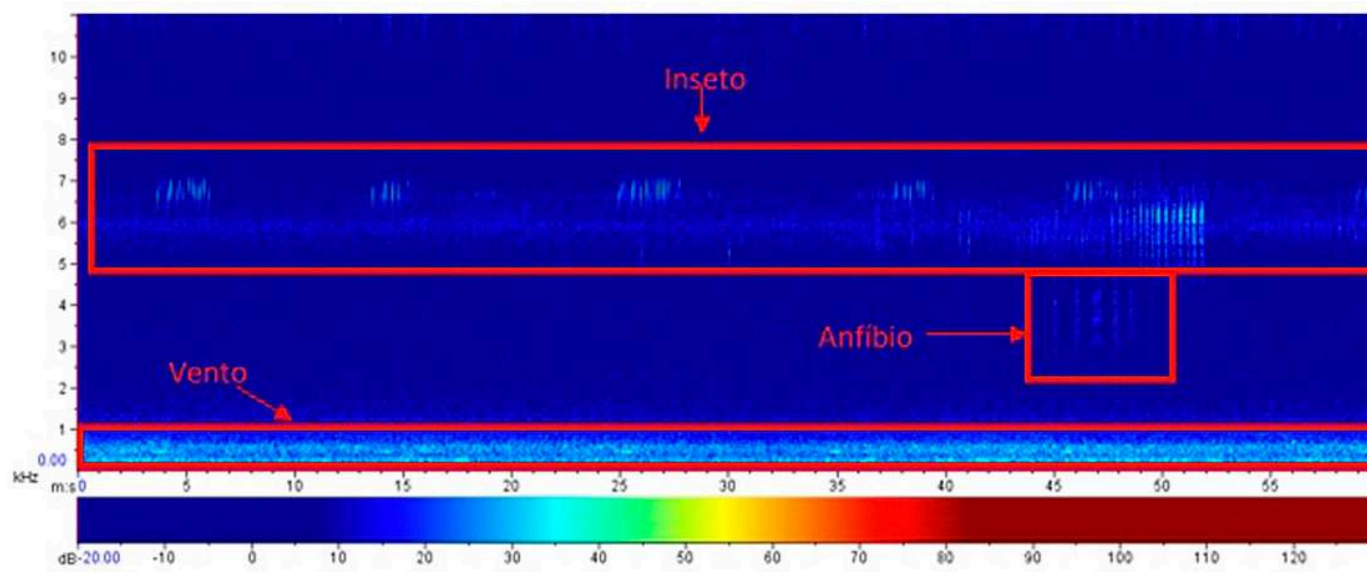
Figura 12. Espectrograma da Restinga do Piano, às 16:35h do dia 16/07/2018 com predominância da biofonia entre 2 e 7,50 kHz. Abaixo encontra-se a escala de cores da Potência (dB)
