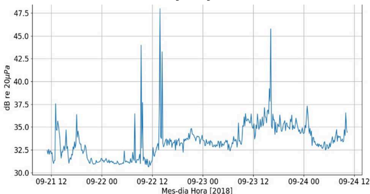
Figura 11. Potência média (y) x mês-dia e hora (x) contendo picos de potência registrados de geofonia e antropofonia no período de 21 a 24 de setembro de 2018, na Restinga do Foguete obtidos na faixa de 0,1 - 1,5 kHz
