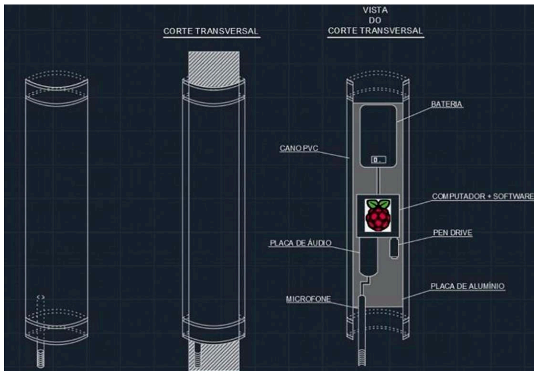
Figura 6. Esquema do EA-1: A primeira imagem apresenta a visão total do equipamento, em seguida a simulação de um corte transversal e por último, a visão interna do equipamento após o corte transversal
