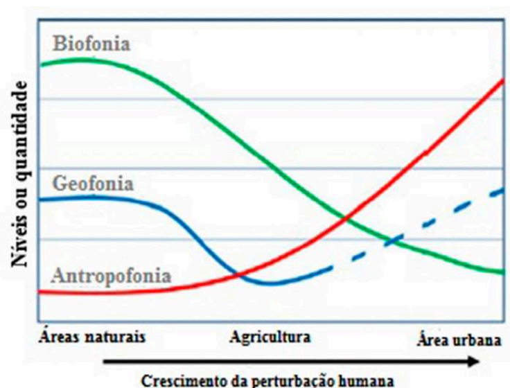
Figura 2. Relação entre os elementos da paisagem acústica, com redução dos níveis de biofonia onde há elevação dos níveis de antropofonia
