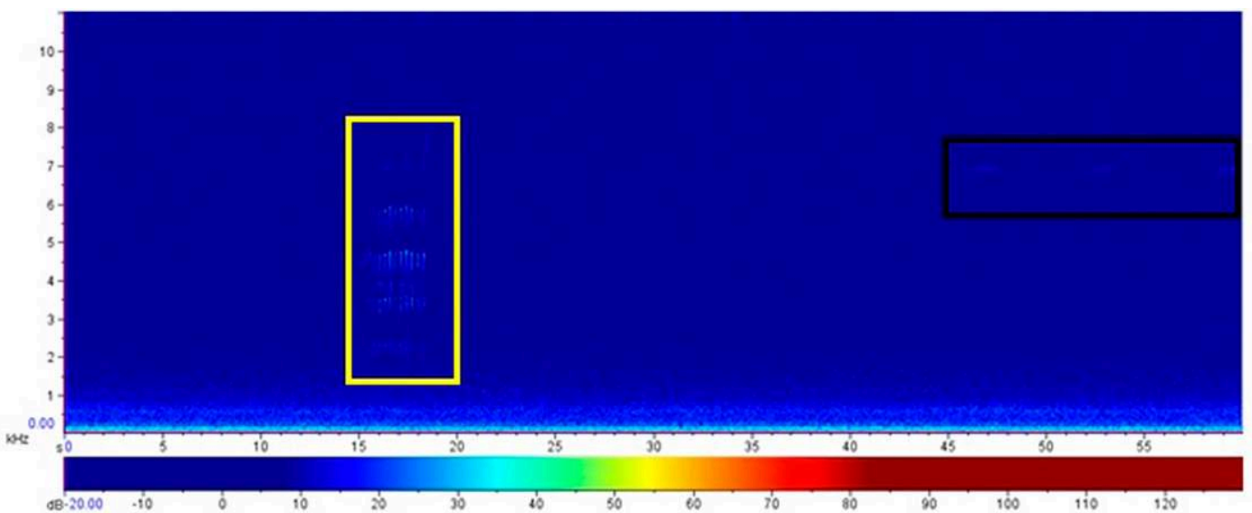
Figura 15. Duas assinaturas bioacústicas às 14:40h do dia 21/09/2018, na Restinga do Foguete. Em amarelo, a biofonia de uma ave e em preto, de um inseto
