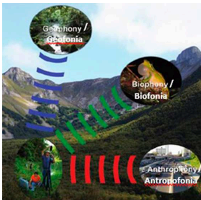
Figura 1. Composição da paisagem acústica
