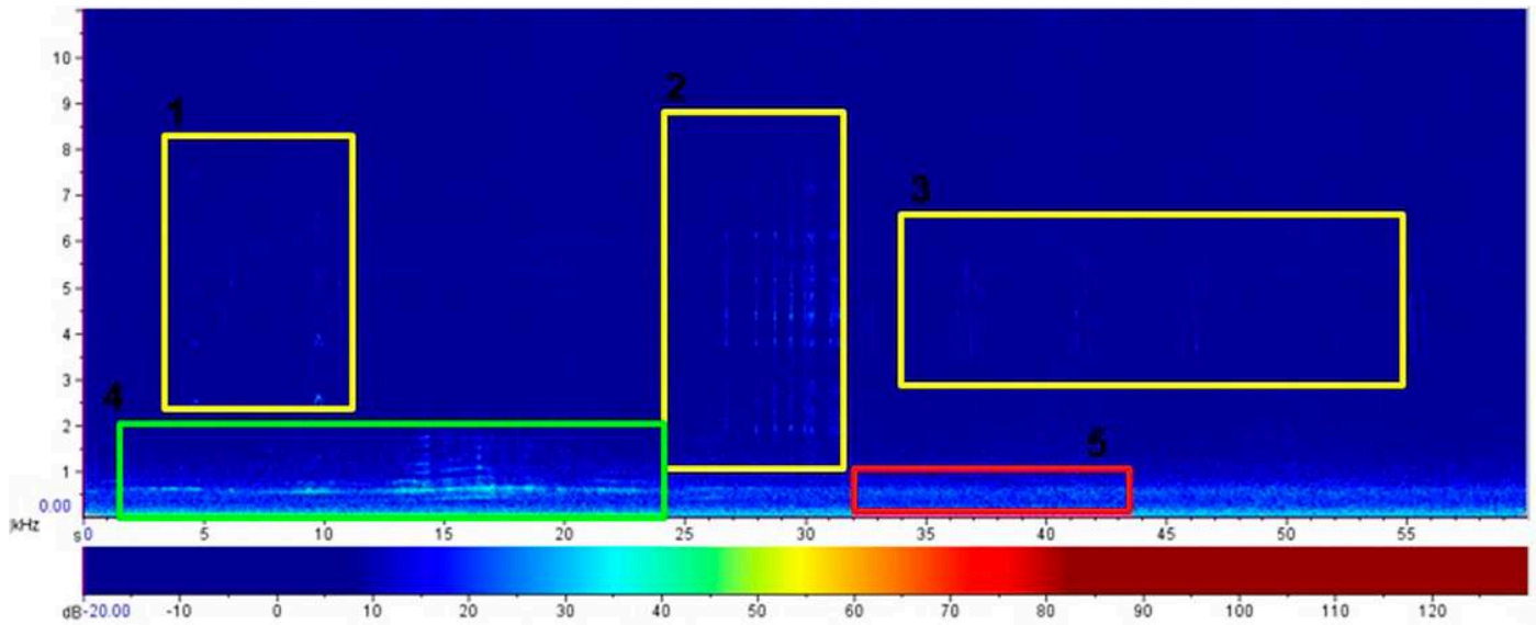
Figura 16. Espectrograma da Restinga do Foguete, às 17:25h do dia 22/09/2018, contendo biofonia nos itens 1, 2 e 3, antropofonia (moto) no item 4 e geofonia (vento) no item 5
