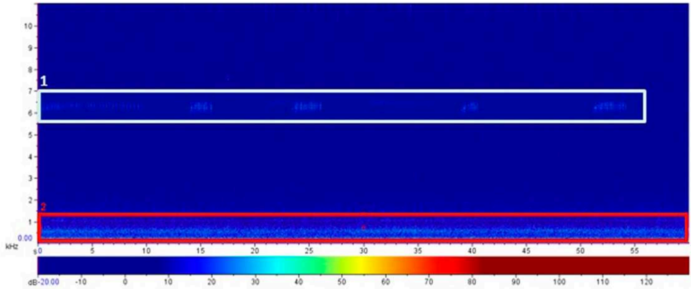
Figura 14. Espectrograma da Restinga do Foguete, às 13:45h do dia 21/09/2018. A faixa superior (1) (entre 5,5 e 8 kHz) apresenta insetos e a faixa inferior (2) (0 a 1,5 kHz) apresenta a geofonia (vento)
