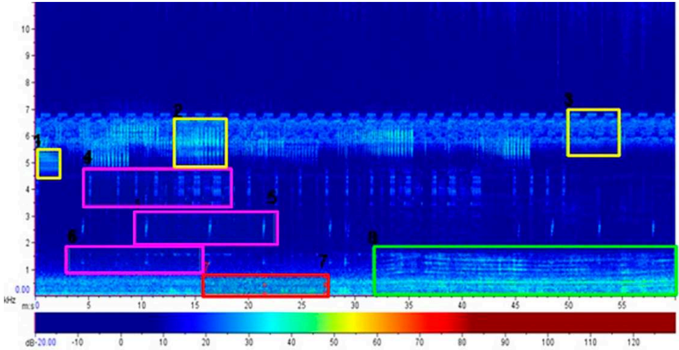
Figura 13. Espectrograma da Restinga do Piano, às 19:50h do dia 16/07/2018, com a escala de cores abaixo. 1, 2 e 3: insetos; 4, 5 e 6: anfíbios; 7: geofonia (vento); 8: antropofonia (motocicleta)
