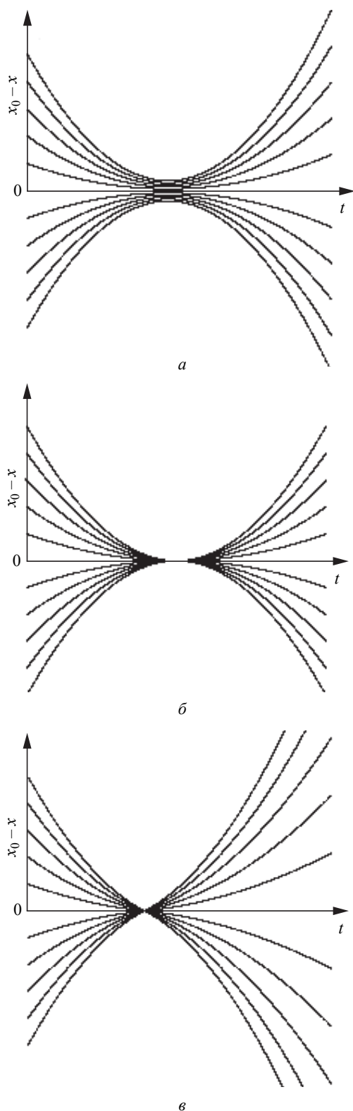
Рис. 5. Групування електронів (у системі координат, яка рухається зі швидкістю робочої гармоніки) у тонкому шарі, коли поздовжній розмір ущільнення можна порівняти із товщиною шару: а – електрони, наблизившись до точки x = x_0 , розходяться; б – електрони зупиняються у точці x = x_0 (оптимальний випадок); в – електрони збираються у точці x = x_0 , але одразу розходяться
