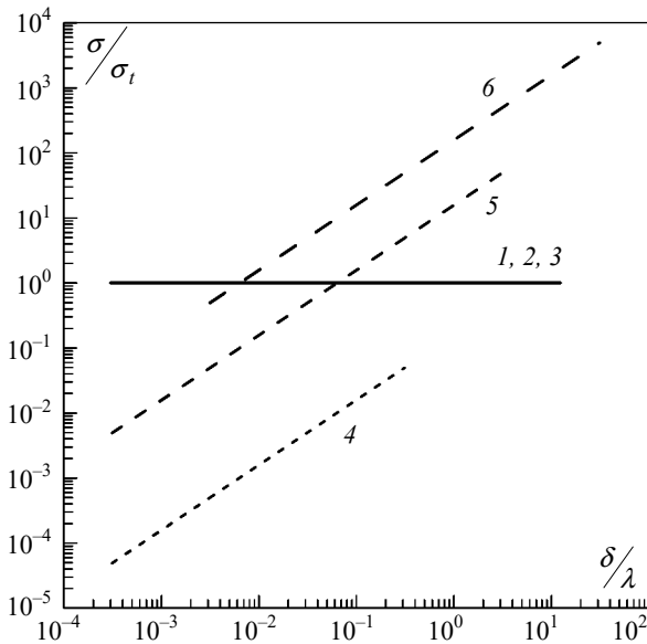
Рис. 4. Нормовані ЕПР абсолютно провідної круглій пластини ( \lambda = 3,2 см) радіусом R_b : криві 1, 4 – R_b = 0,1 м; криві 2, 5 – R_b = 1 м; криві 3, 6 – R_b = 10 м
