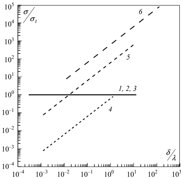
Рис. 5. Нормовані ЕПР абсолютно провідної круглій пластини ( \lambda = 8 мм) радіусом R_b : криві 1, 4 – R_b = 0,1 м; криві 2, 5 – R_b = 1 м; криві 3, 6 – R_b = 10 м
