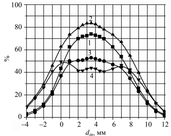
Рис. 11. ЗДДР с ЭС – отверстием в диафрагме. Фактор нерезонансных потерь: 1 – \varnothing 2,6 мм; 2 – \varnothing 3,1 мм. Эффективность возбуждения: 3 – \varnothing 2,6 мм; 4 – \varnothing 3,1 мм
