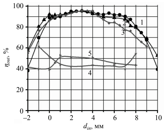
Рис. 7. Эффективность вывода ЗДДР: со щелевыми ЭС (1 – 0,3×7,2 мм; 2 – 0,6×7,2 мм; 3 – 0,6×7,2 мм; измерено методом баланса мощностей); с ЭС в виде отверстий в диафрагме (4 – Ø2,6 мм; 5 – Ø3,1 мм)
