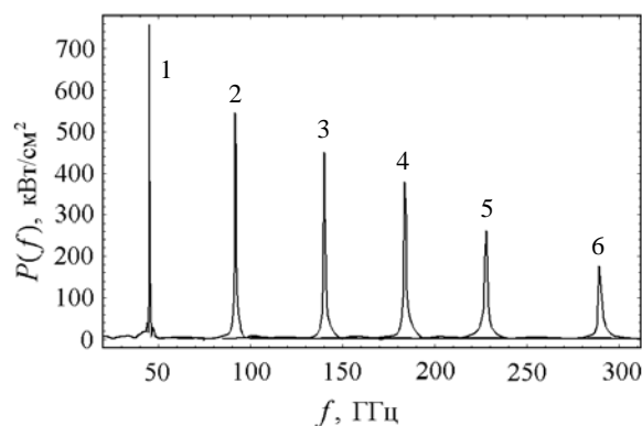
Рис. 8. Фурье-спектр плотности выходной мощности P(f) шести вариантов Si ЛГД в режиме когерентных двухчастотных автоколебаний
