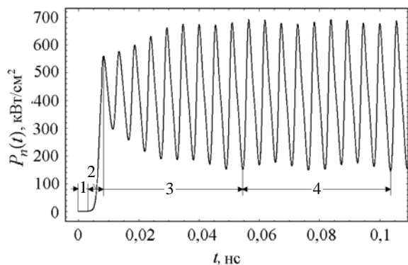
Рис. 7. Динамика развития и установления автоколебаний электронной компоненты плотности мгновенной мощности P_n(t) когерентного Si ЛГД
