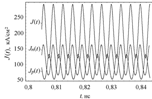
Рис. 6. Зависимости от времени электронной J_n(t) и дырочной J_p(t) компонент плотности лавинного тока J(t) когерентных Si ЛГД
