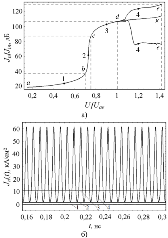
Рис. 1. Статическая ВАХ ЛГД на основе резкого GaAs p-n -перехода (а) и зависимость от времени электронной компоненты плотности лавинного тока J_n(t) в различных точках ВАХ (б). Кривые 1–4 соответствуют точкам 1–4 ВАХ
