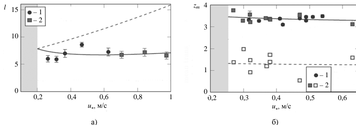
Рис. 6. Расчетные и экспериментальные зависимости средней длины прыжка частиц (а) и средней высоты слоя частиц в потоке эоловой транспортировки от скорости сдвига (б)
