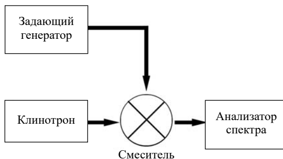
Рис. 4. Схема детектирования электромагнитного излучения клинотрона и измерения частоты генерации при помощи спектроанализатора
