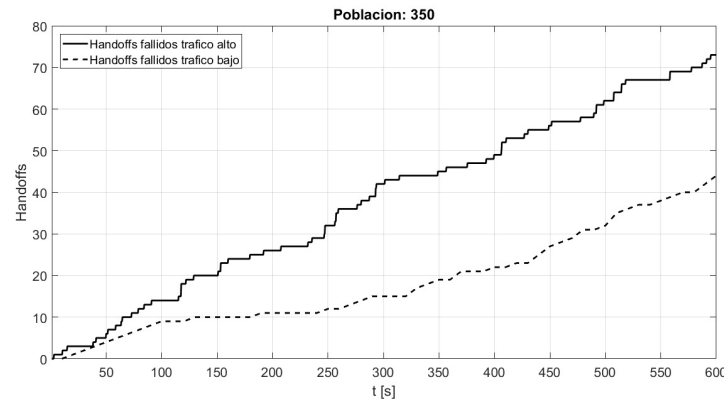
Figura 5. Resultados método propuesto para una población de 350 Fuente: elaboración propia.
