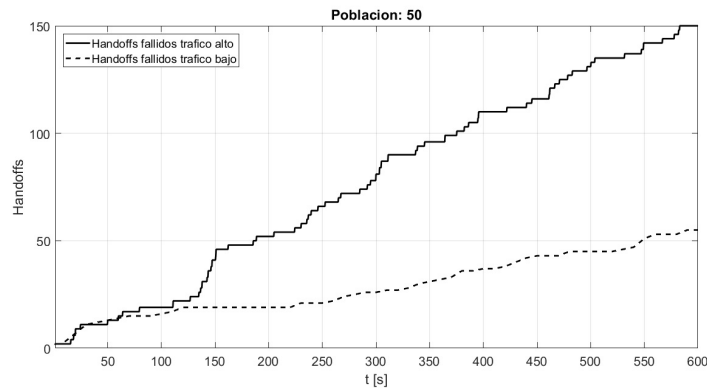
Figura 2. Resultados método propuesto para una población de 50 Fuente: elaboración propia.
