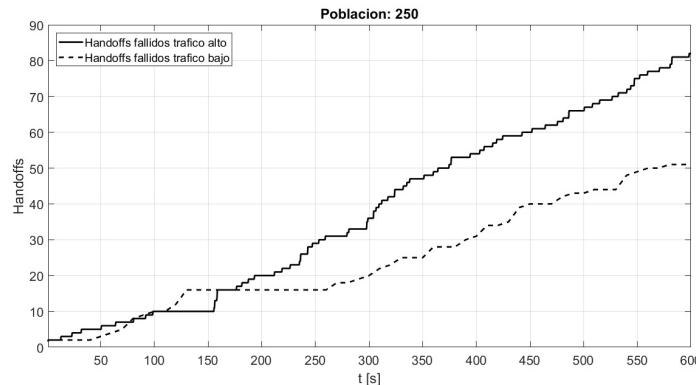
Figura 4. Resultados método propuesto para una población de 250 Fuente: elaboración propia.
