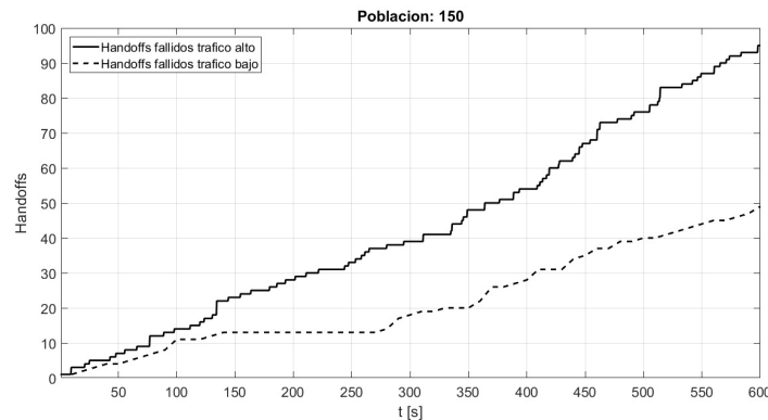
Figura 3. Resultados método propuesto para una población de 150 Fuente: elaboración propia.
