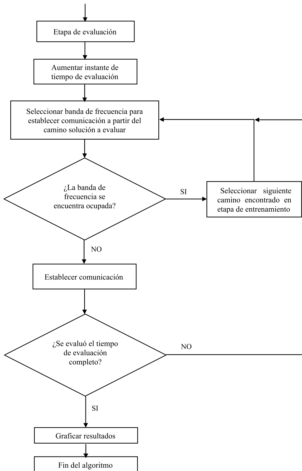
Figura 1. Diagrama de flujo del algoritmo propuesto Fuente: elaboración propia.
