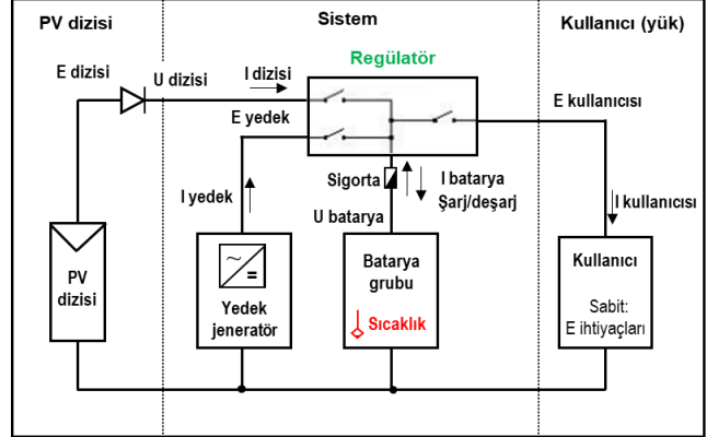
Şekil 1: 1 kW tipik bir çatı tip şebekeden bağımsız FV sisteminin şematik gösterimi.
