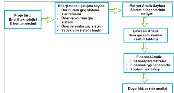
Şekil 3: RETScreen platformu: Altı adımlı standart analiz akış diyagramı.
