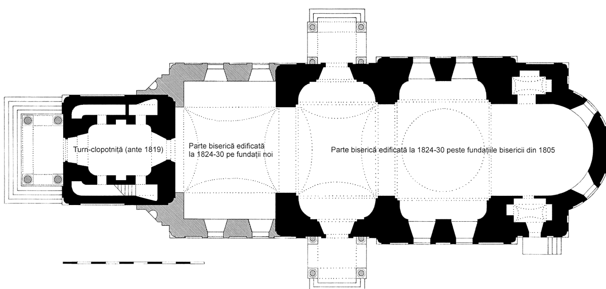
Fig. 4. Biserica Înălțarea Domnului (1830). Plan (de S. Ciocanu).
