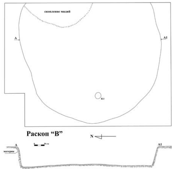
Рис. 6. Викторовка-I. Раскоп «В». Земляночное жилище № 1. План и разрез.
