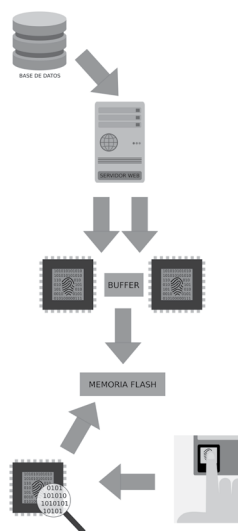
Figura 11. Proceso de autenticación con modificaciones al proceso estándar.
