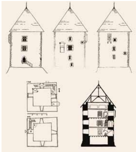
Slika 7. Rekonstrukcija središnje kule/palasa (crtao: Zorislav Horvat, 1995. – 2009.)
