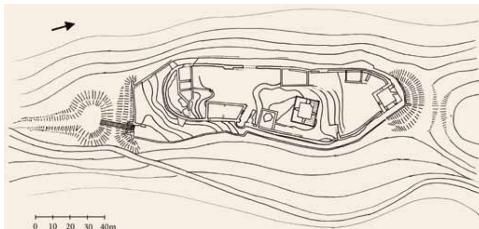
Slika 9. Plemićki grad Garić, situacija, skica (crtao: Krešimir Regan, 2010.)
