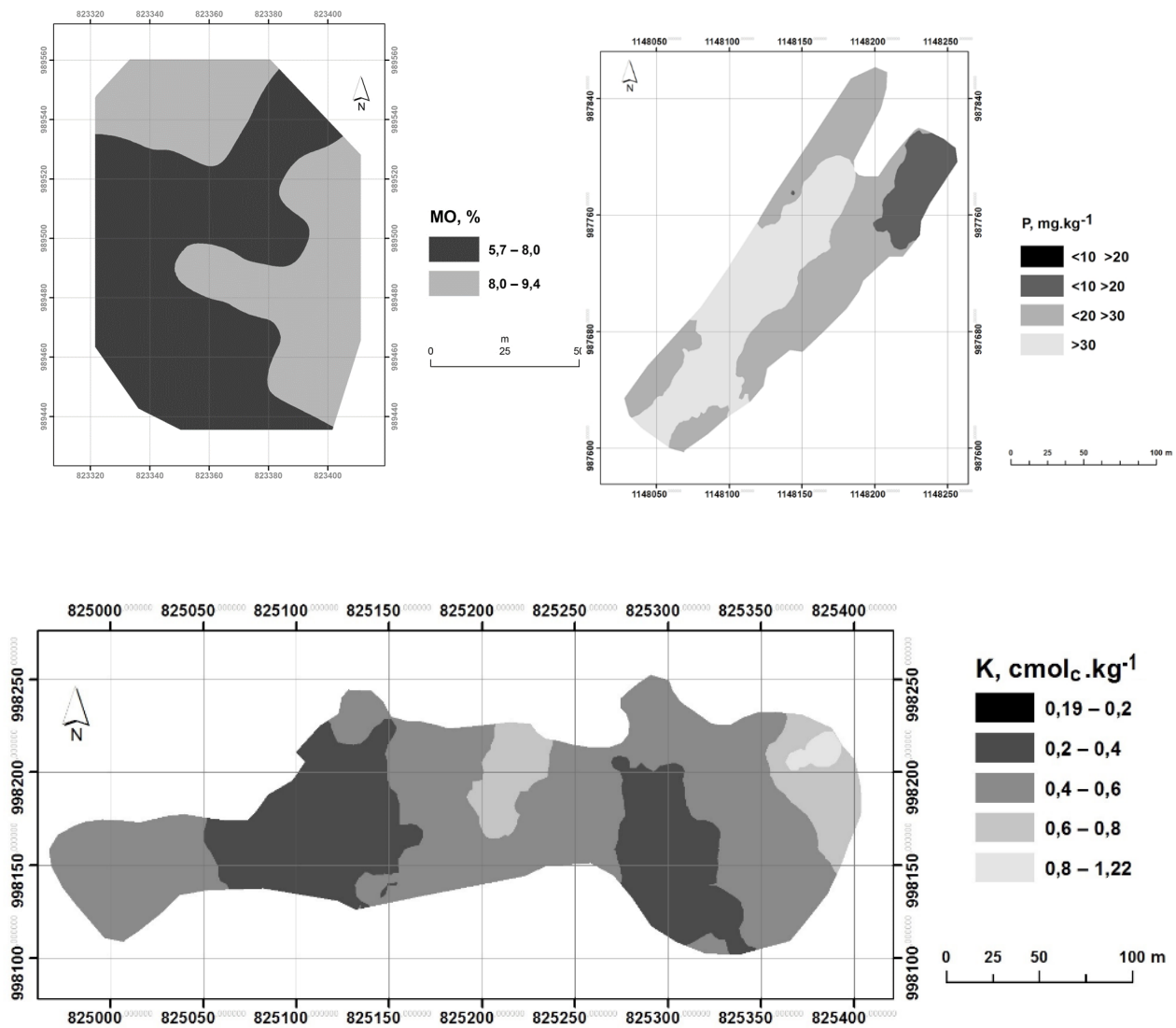
Figura 7. Mapas de variabilidad para MO (%) en el lote de 1,0 ha; P ( \text{mg.kg}^{-1} ) en el lote de 2,0 ha; K ( \text{cmol}_c.\text{kg}^{-1} ) en el lote de 3,5 ha.
