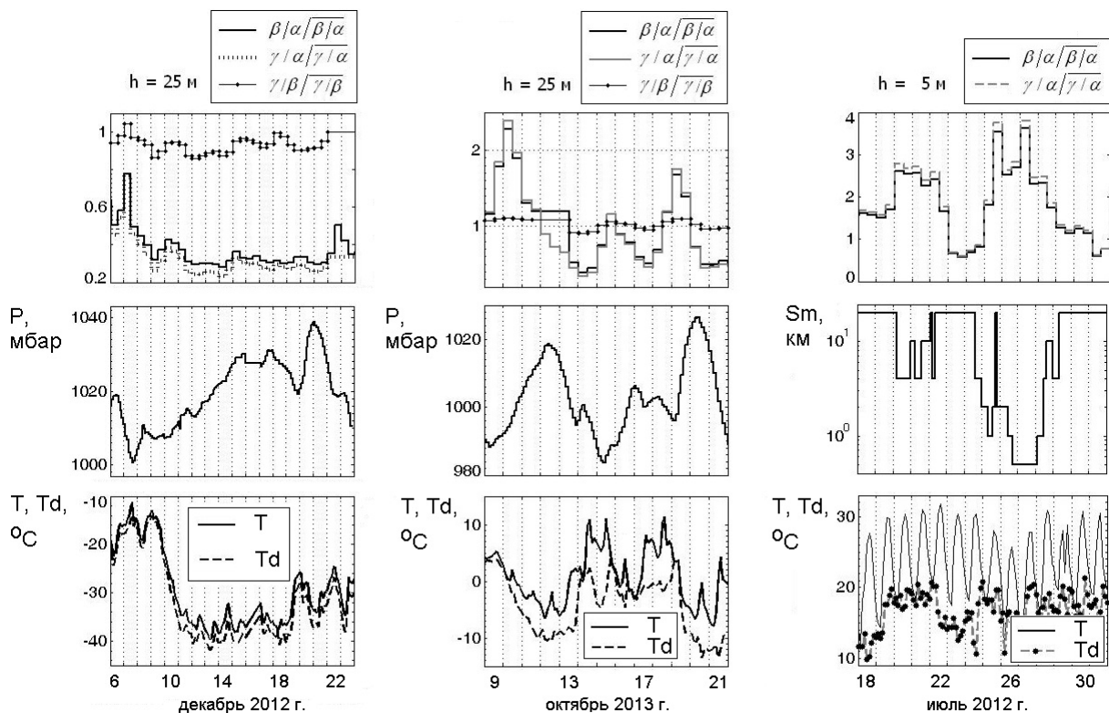
Рис. 5. Реакция трассеров-индикаторов на экстремально низкие температуры и экстремально высокое атмосферное давление (а), прохождение серии циклонов (б), задымленность атмосферы от интенсивных летних лесных пожаров (в). Здесь: T_d – температура точки росы, S_m – дальность видимости, h – высота расположения сцинтилляционных датчиков. Интервалы усреднения: данных по ионизирующим излучениям – одни сутки; метеоданных – 3 часа
