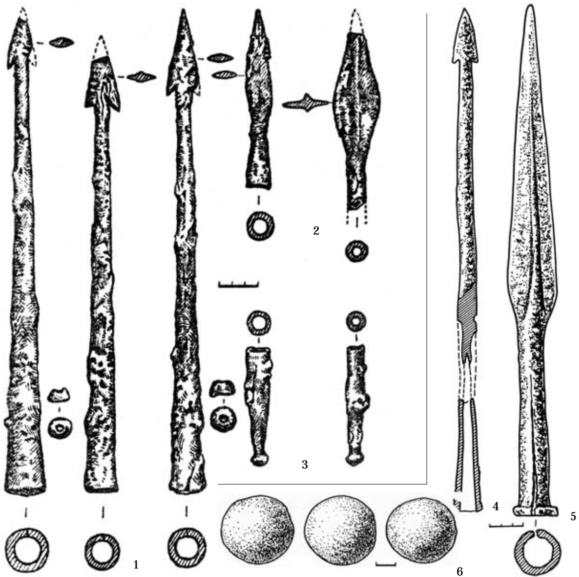
Рис. 4. Оружие из курганов амазонок: наконечники дротиков (1, 4) и копий (2, 5), подтоки (3), пращевые камни (6). 1-3 курган 13 Стеблевского могильника; 4-6 - курган 5 у с. Зеленое. 1-5 - железо, 6 - камень.
