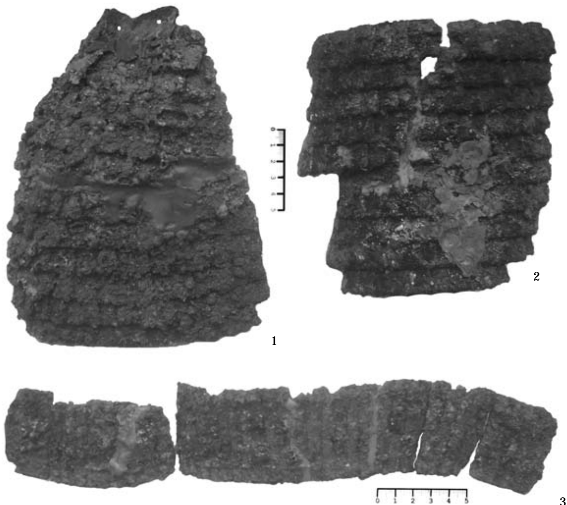
Рис. 6. Детали доспеха из кургана 5 у с. Зеленое.
