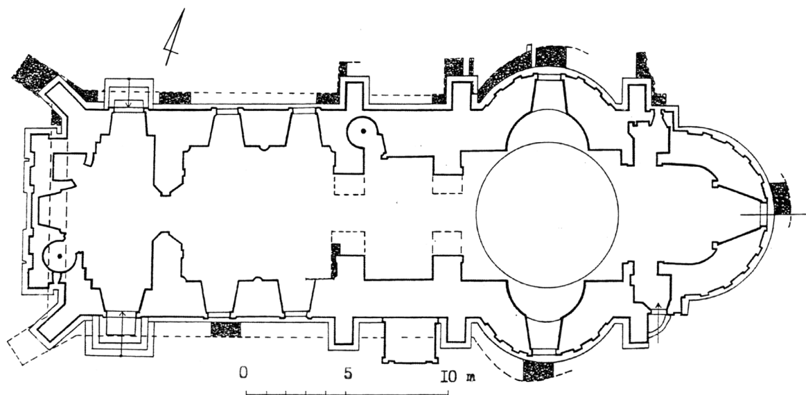
Fig. 7. Planul bisericii Adormirea după săpăturile arheologice (apud Postică, Constantinescu 1996).
