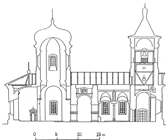
Fig. 3. Secțiunea longitudinală a bisericii Adormirea.
