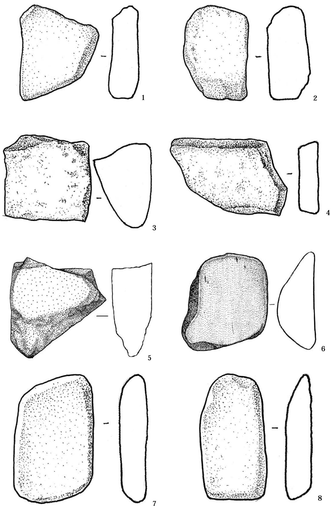
Fig. 1. Răzuitoare din piatră: 1, 2, 7, 8 - Odaia-Miciurin (după Sava, Kaiser 2004, fig. 16/7, 63/2; Sava 2008, fig. 16/7, 24/5); 3, 4 - Căușeni (după Левинский 1986, рис. 8/1, 3); 5 - Petrușeni (după Sava 1992, fig. 6/1); 6 - Cobâlea (după Левицкий 1988, рис. 28/1).
