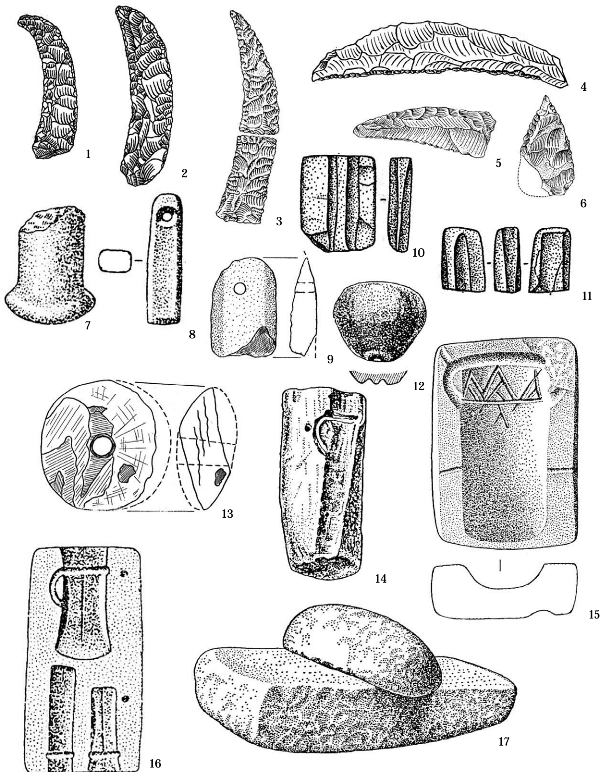
Fig. 11. Unelte din piatră și din silex descoperite în cadrul unor culturi sincronice sau parțial sincronice complexului cultural Noua-Sabatinovka. Culturile: Komariv (1, 2, 10, 11, 13), Gava-Holigrady (4, 9), Belogradovka (3, 5, 6, 12, 14), Belozerka (7, 8, 16), Srubnaja (15, 17). 1-5 - cuțite; 6 - vârf de săgeată; 7 - sceptru/pisălog; 8, 9 - cute; 10, 11 - polizoare; 12 - măciucă; 13 - fusaiolă; 14-16 - forme de turnat; 17 - rășniță. 1, 2, 10, 11 - Coteala; 3 - Kirovo; 4, 9, 13 - Miškovič; 5 - Belogradovskij Les; 6, 14 - Sobkovka; 7 - Uškalka; 8 - Zapovitne; 12 - Andrusovka; 15 - Plipečatino; 16 - Zavadovka; 17 - Iličovka. 1, 2, 10, 11 (după Sava 1994, fig. 3/19, 20, 30, 33); 3, 5-8, 12, 14-17 (după Археология 1985, рис. 112/40; 127/1, 20; 136/1, 4, 5, 7; 142/19, 44, 52); 4, 9, 13 (după Малеев 1976, рис. 2/7, 10, 11).
