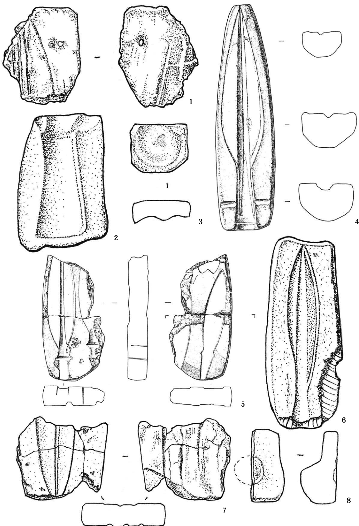
Fig. 7. Forme de turnat din piatră: 1 - Cobălea (după Левицкий 1988, рис. 27/1); 2, 6 - Ostrivec' (după Археология 1985, рис. 131/32, 36); 3, 8 - Odaia-Miciurin (după Сава, Кайзер 2011, рис. 88/2, 4); 4, 5 - Bălănești (după Sava 2011, Abb. 5/1, 6/1); 7 - Mahala (după Смирнова 1972, 24, рис. 9/1).
