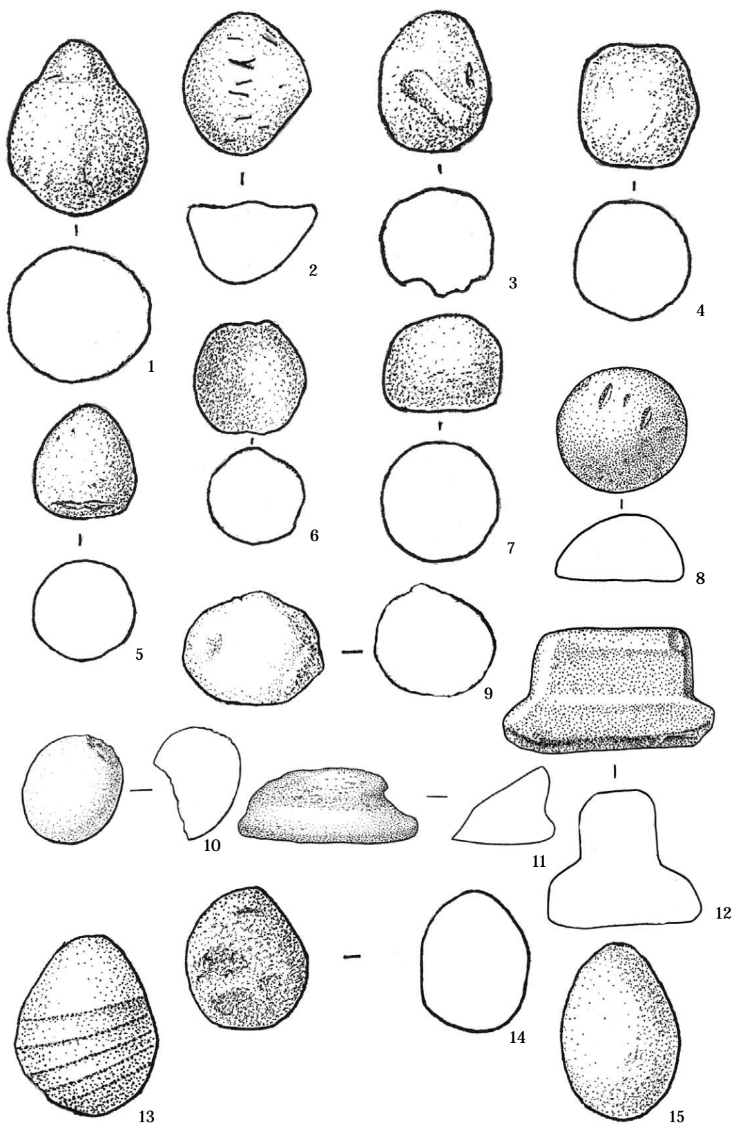
Fig. 5. Șlefuitoare-lustruitoare: 1-5, 7, 10, 11 - Odaia-Miciurin (după Сава, Кайзер 2011, рис. 87/3-6, 9, 13); 6 - Nisporeni; 8 - Căușeni (după Левинский 1986, рис. 8/2); 9 - Cobălea (după Левицкий 1988, рис. 18/6); 12 - Ghindești (după Мелюкова 1958, табл. XXVI/8). Percutoare din piatră: 10, 14 - Odaia-Miciurin (după Сава, Кайзер 2011, рис. 87/14, 15); 13 - Ghindești (după Мелюкова 1957, табл. XIX/5); 15 - Novoselicja (după Тоцев, Черняков 1986, рис. 6/11).
