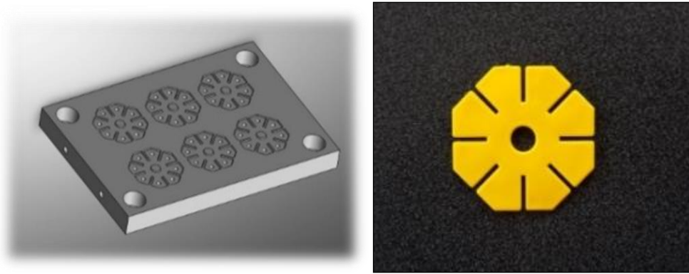
Figura 1. Roseta plástica y molde seis cavidades de acero
