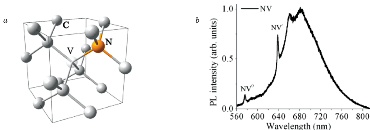
Рис. 8. Схематичне зображення центру нітрогенвакансії — NV (нітроген показано жовтим): а — дефект може існувати у двох станах заряду: нейтральному NV^0 та негативно зарядженому NV^- ; б — флуоресценція діаманта. Максимуми флуоресценції центрів нітрогенвакансії позначено NV^0 (575 nm) та NV^- (637 nm); лінії фонів — PL [100]
