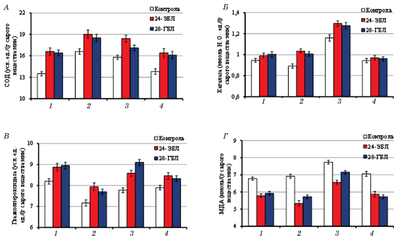
Рис. 2. Активность СОД (А), каталазы (Б), гваяколпероксидазы (В) и содержание МДА (Г) в этилированных проростках пшена при действии БС и повреждающего прогрева:
