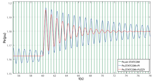
Figura 19. Respuesta de P_e en sobrecarga ante un aumento del 1.5% en la potencia mecánica
