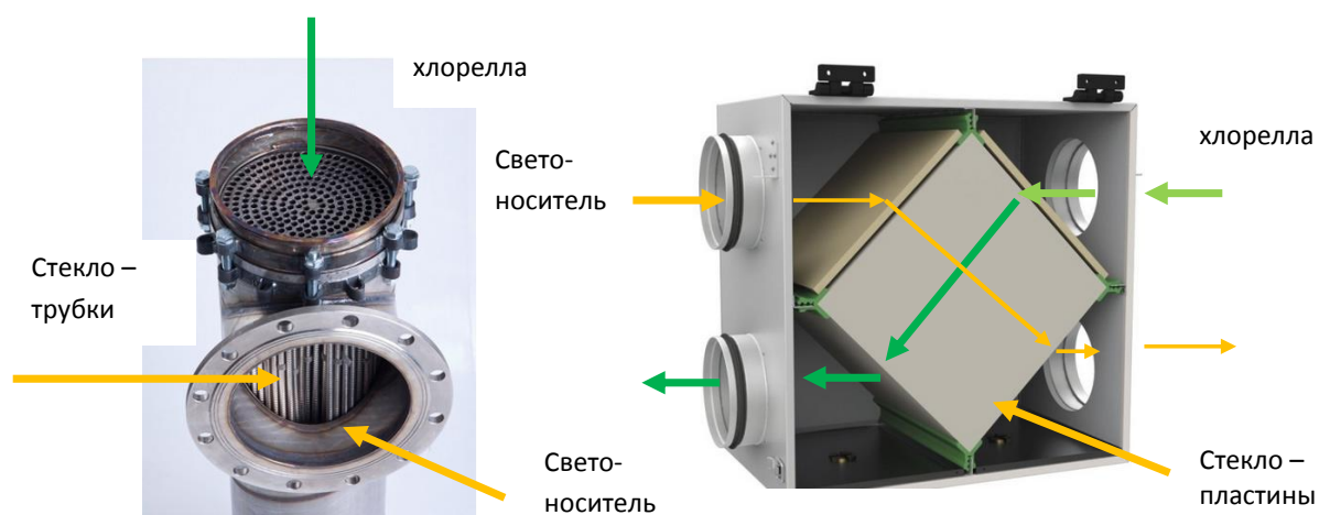
Рис. 11. Констр. Рис. 11 ообменника
