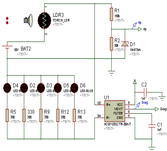
Рис. 6. Диаграмма моделирования цепи измерения напряжения и тока
