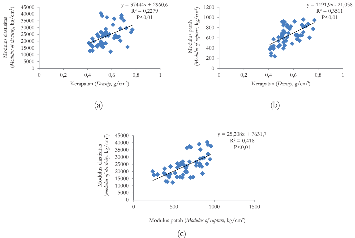
Gambar 2. Korelasi antara kerapatan dengan modulus elastisitas (a), kerapatan dengan modulus patah (b), dan modulus patah dengan modulus elastisitas (c) Figure 2. Corelation between density and modulus of elasticity (a), density and modulus of rupture (b), modulus of rupture and modulus of elasticity (c)
