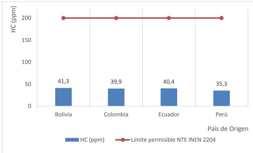
Figura 4. Emisiones de hidrocarburos (Prueba rpm altas)
