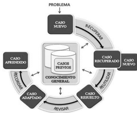
Figura 1: Ciclo Razonador Basado en Casos. (Cordero Morales et al., 2013)
