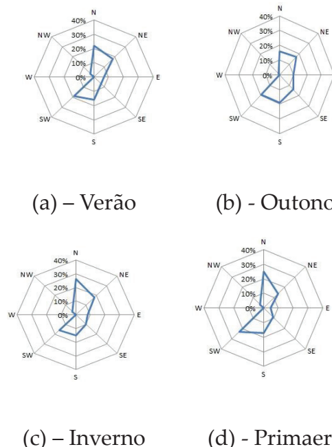
Figura 5 – Distribuição sazonal de frequência das direções predominantes do vento na estação automática do IFSC, no período de 2004 a 2012
