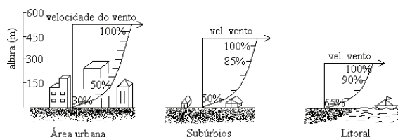
Figura 2 - Variação do vento com a altura Fonte: FERREIRA & LEITE, 2006
