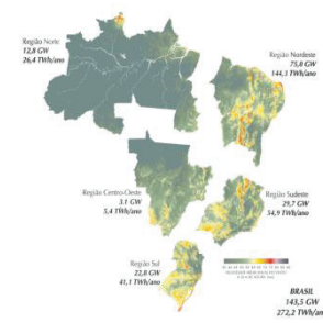
Figura 1 - Velocidades médias anuais do vento à 50 m de altura e potencial eólico Fonte: Atlas do Potencial Eólico Brasileiro, 2001
