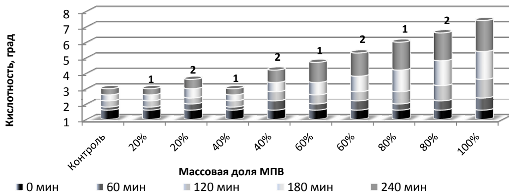
Рис. 2. Влияние массовой доли МПВ и стадии ее внесения на кислотонакопление в опаре, где 1 – 1 способ, 2 – 2 способ
