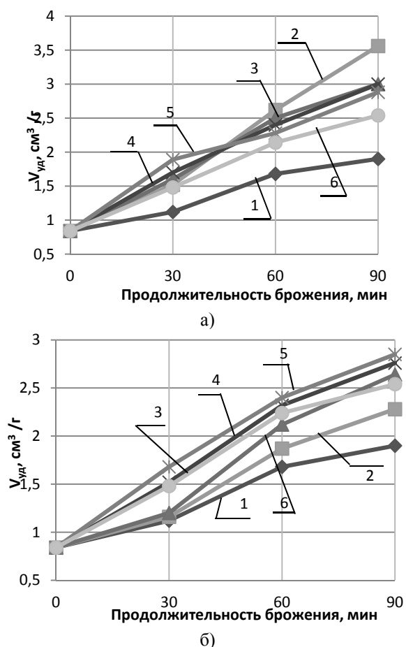
Рис. 4. Изменение удельного объема кексового теста при брожении (а – 1 способ, б – 2 способ), где массовая доля МПВ (%): 1 – 0; 2 – 20; 3 – 40; 4 – 60; 5 – 80; 6 – 100
