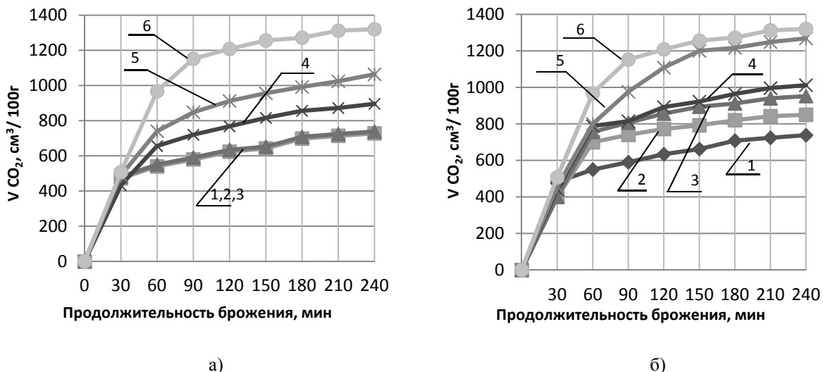
Рис. 1. Количество выделенного углекислого газа при брожении опары (а – 1 способ, б – 2 способ), где массовая доля МПВ (%): 1 – 0; 2 – 20; 3 – 40; 4 – 60; 5 – 80; 6 – 100
