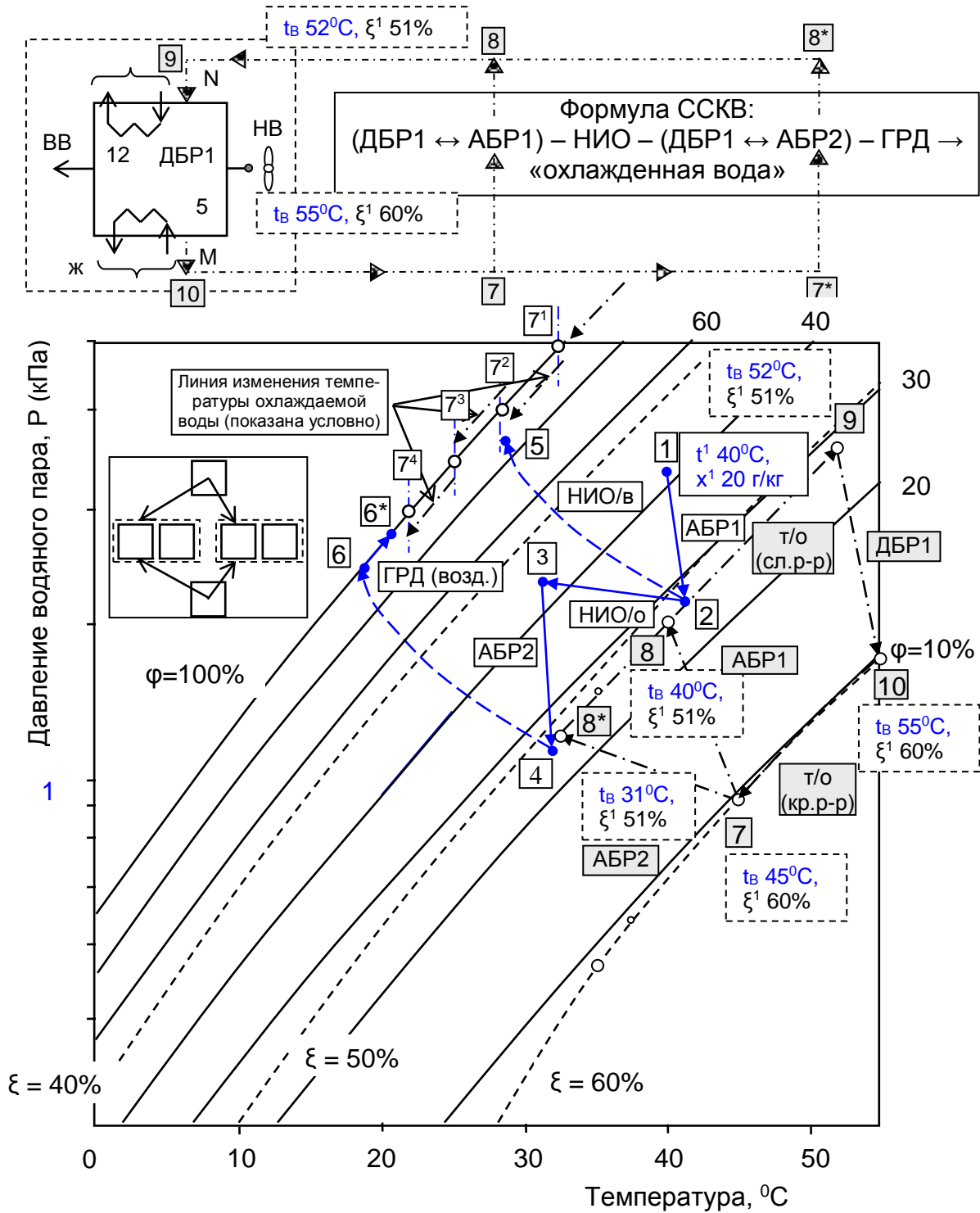
Рисунок 2 – Изображение процессов в СХС на совмещенной диаграмме р-Т для раствора LiBr+ – влажный воздух (формула АБР1-НИО1-АБР2-ГРД, схема по рис. 1А, НВ: t^1 40^\circ\text{C} , x^1 20 \text{ г/кг} ).
