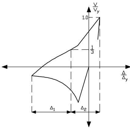
Şekil 18: \Delta_1 ve \Delta_2 tanımları (Lee ve Goel [25]'den uyarlanmıştır) [26].
