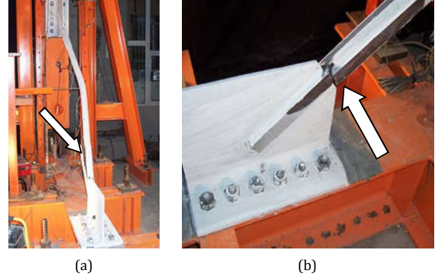
Şekil 13: TB-2 numunesinin, (a): -4\delta_y ’de burkulması ve CFRP plakasının çelik yüzeyden ayrılması, (b): Alt uç kesitten kopma.
