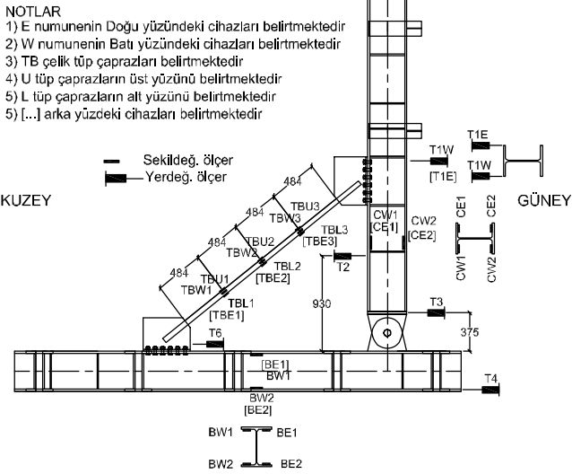
Şekil 9: şekildeğiştirme ve düzlem içi yerdeğiştirme ölçerlerin yerleşimi.
