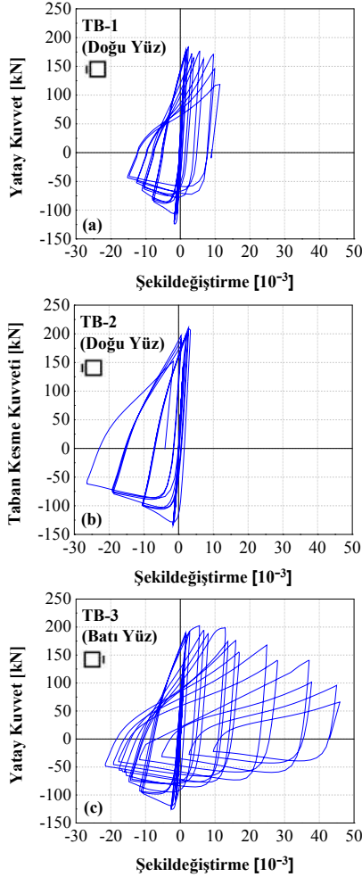
Şekil 21: (a): TB-1, (b): TB-2, (c): TB-3 numunelerinin orta bölgelerindeki taban kesme kuvveti-şekildeğiřtirme eđrileri.
