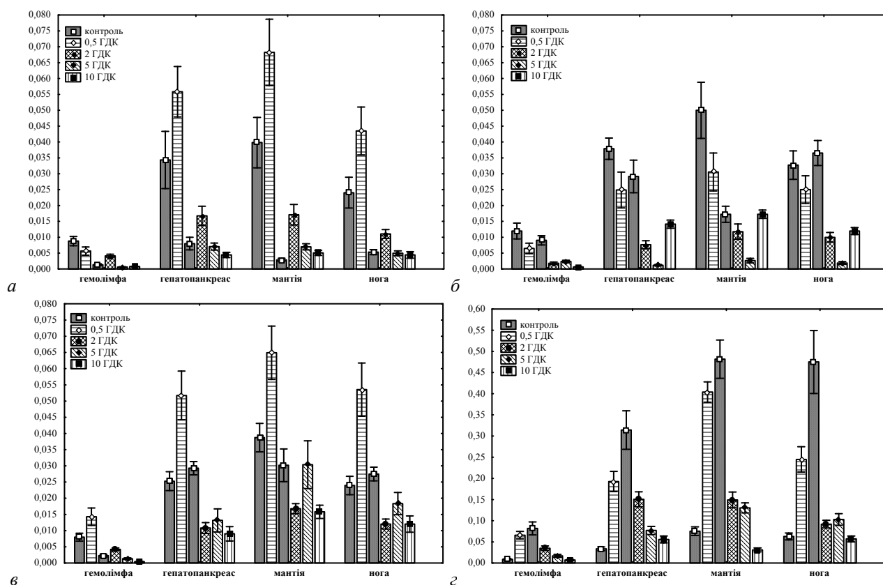
Рис. 1. Вплив амоній хлориду (0,5–10 ГДК) на вміст \beta -каротину в організмі L. stagnalis : а – експозиція 2 доби, б – 7 діб, в – 14 діб, з – 21 доба; по осі абсцис – тканини (органи) моллюсків, по осі ординат – вміст \beta -каротину (мг/г сирової тканини); n = 10 для кожного варіанта досліджу
