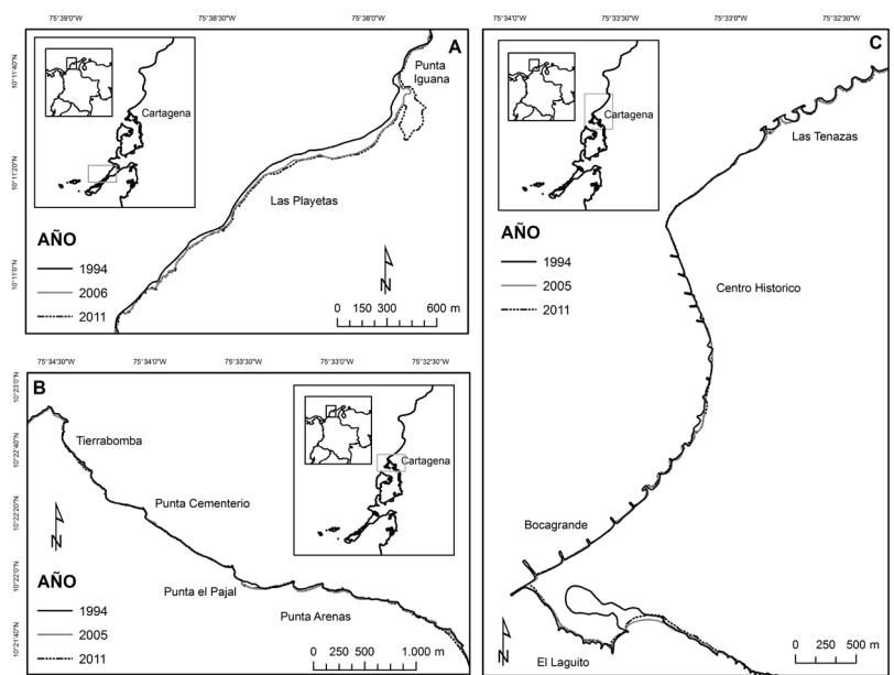
Figura 2. Mapa de cambios en la línea de costa en los sectores de a) Playetas, b) Tierrabomba y c) Cartagena de Indias.
