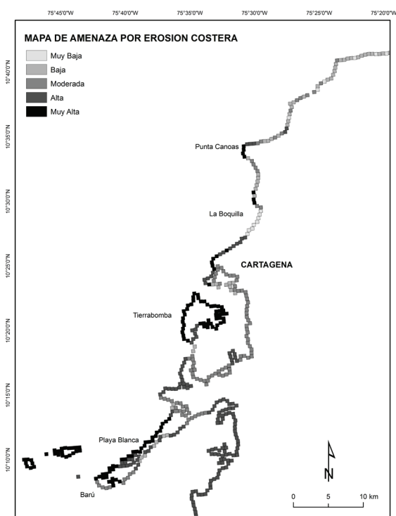
Figura 4. Mapa de amenaza por erosión costera en el área de estudio (Tomado de INVEMAR-MADS, et al., 2012).
