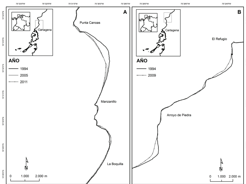
Figura 3. Mapa de cambios en la línea de costa en los sectores de a) La Boquilla y b) Sector norte del área de estudio.
