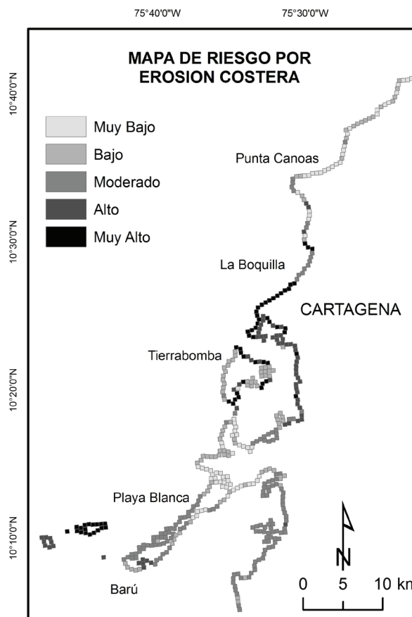
Figura 7. Mapa de riesgo por erosión costera para la línea de costa del área de estudio (Tomado de INVEMAR-MADS, et al., 2012).
