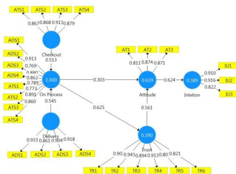
Gambar 2 Model fit faktor sikap dan faktor perilaku atas penggunaan sistem informasi akademik
