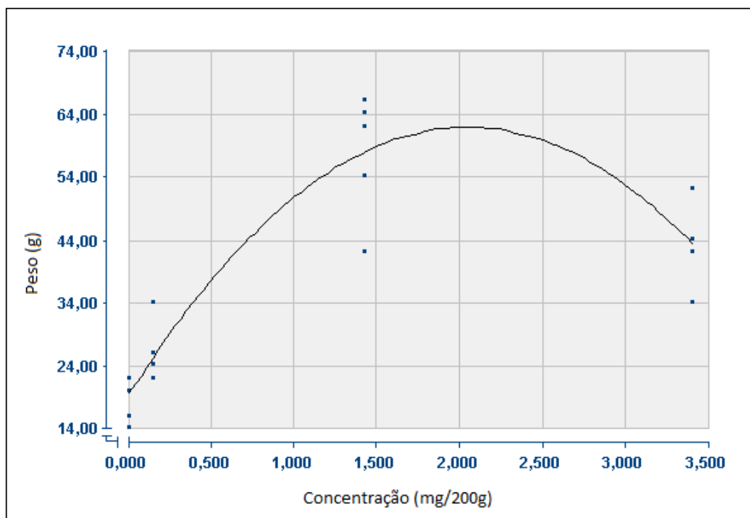
Figura 4: Regressão no modelo quadrático, com valor do peso em função da concentração de Decanoato de nandrolona.
