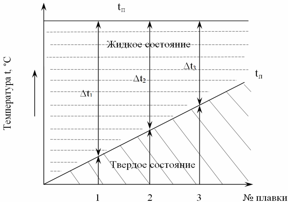
Рис. 1 – Схема различных величин при плавке металла в ванне печи: t_п – температура в печи, обусловленной ее тепловой мощностью; t_{л1} , t_{л2} , t_{л3} - температуры ликвидус отдельных марок сталей; \Delta t_1 , \Delta t_2 , \Delta t_3 – фактический перегрев расплава над линией ликвидус
