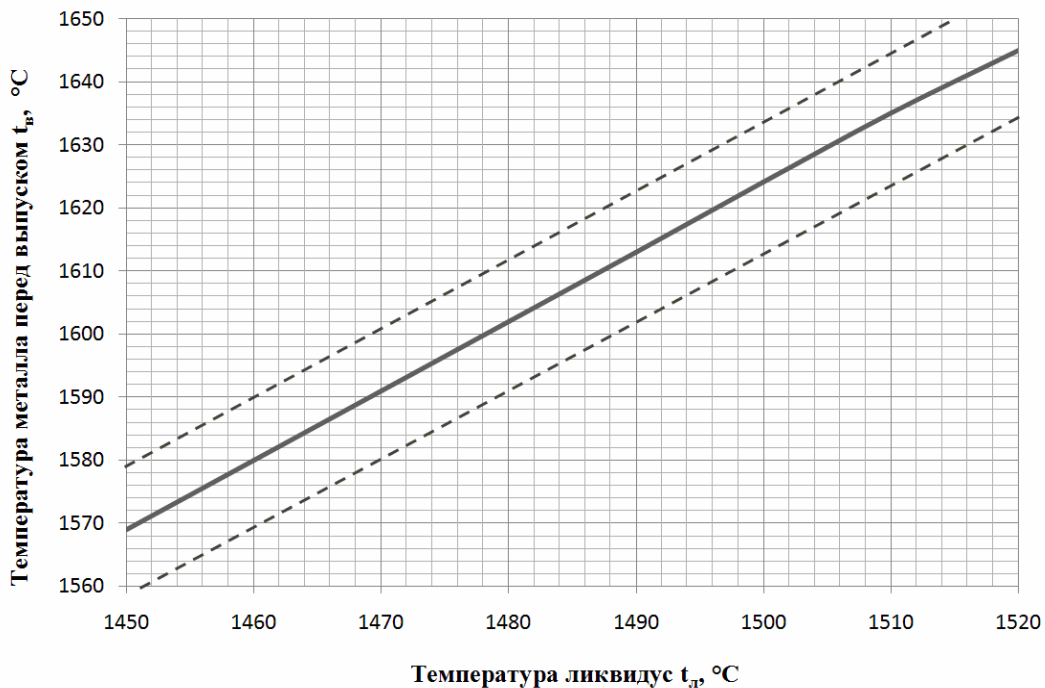
Рис. 3 – Рекомендуемые оптимальные температуры жидкой стали перед выпуском ее из печи в зависимости от температуры ликвидус, ^\circ\text{C} выплавляемой стали
