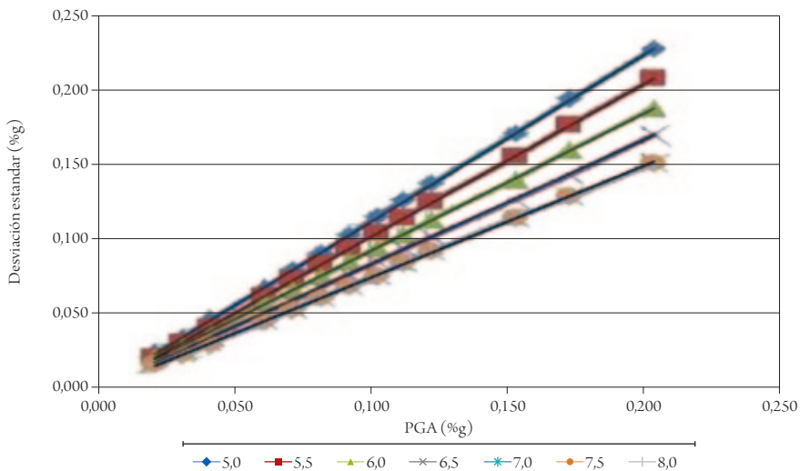
Figura 1. Variación de la desviación estándar como función de la PGA, de la magnitud y de la distancia (modelo AS08)
