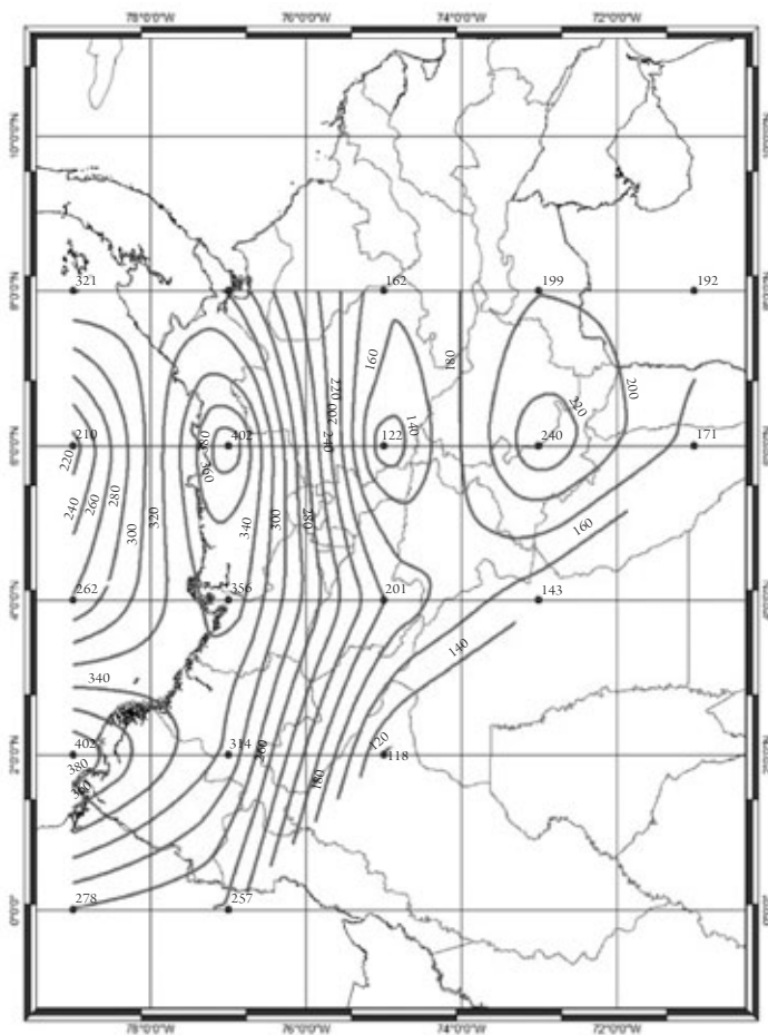
Figura 8. Curvas de isoaceleración para Colombia (modelo I08)
