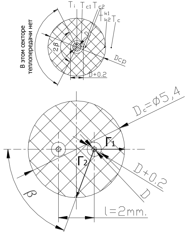
Рисунок 3 – Чертеж керамического (корунд) стержня (2-х канальная соломинка) в котором коаксиально размещены ВТСП проводники с газовым зазором (0.2 мм).
