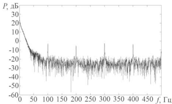
Рис. 5. Спектр тока в рабочей цепи стрелочного электропривода постоянного тока при переводе исправной одиночной стрелки
