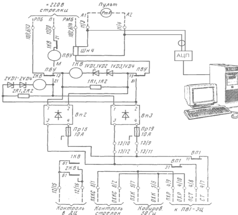
Рис. 1. Подключение измерительного устройства к схеме распределения питания по основным нагрузкам ЭЦ и включения основных приборов панели ПР-ЭЦ
