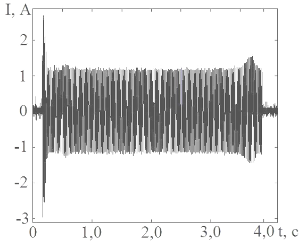
Рис. 11. Ток в рабочей цепи стрелочного электропривода переменного тока при переводе одиночной стрелки с упором корня остряка
