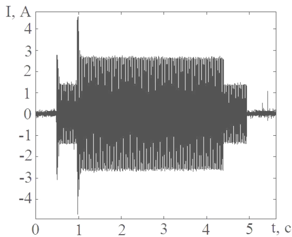
Рис. 14 Ток в рабочей цепи стрелочного электропривода переменного тока при переводе одиночной стрелки с люфтом в шарнирных соединениях и изгибом рабочей тяги
