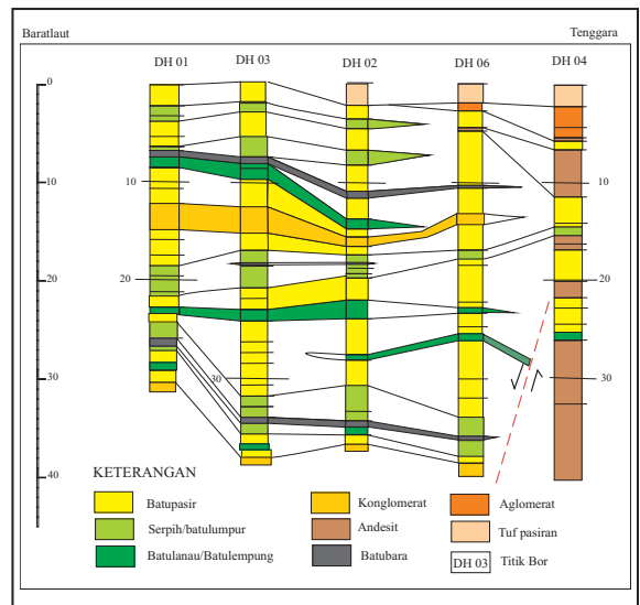
Gambar 14. Korelasi titik bor DH-2-3-4-6 di Lembah Saptajaya.
