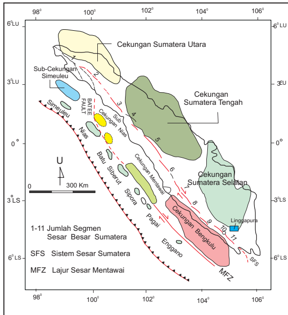
Gambar 2. Posisi Linggapura dalam tataan tektonika dan Cekungan Sumatra Selatan (modifikasi dari Gafoer, 1985; Pulungono, 1985).
