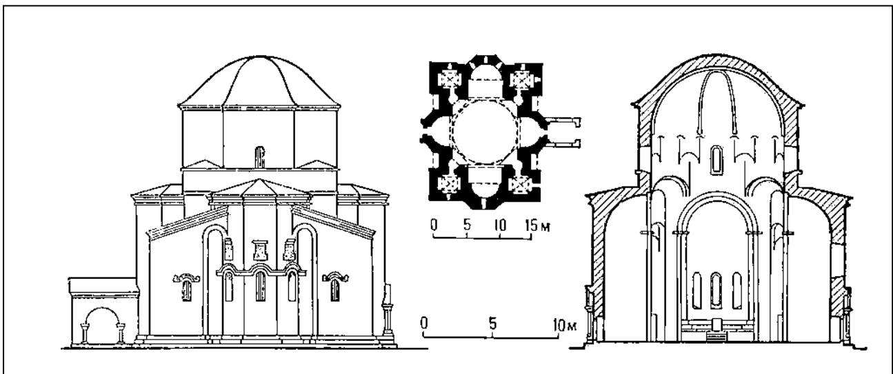
Схема 1. Крестово-купольный тип храма. (Храм Джвари близ Мцхеты, Грузия. Слева направо: фасад, план, разрез.)
