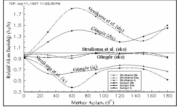
Şekil 4. Kıvrımın kenarlarından 0.2 b kadar içerideki bir hat boyunca ve akım ekseninde akımın etkisiyle oluşan taban şekli
