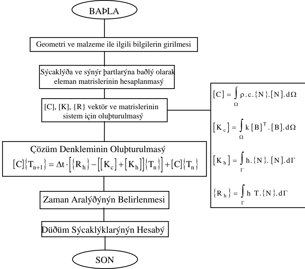
EK-1. Bilgisayar Programı Akıř Őeması
