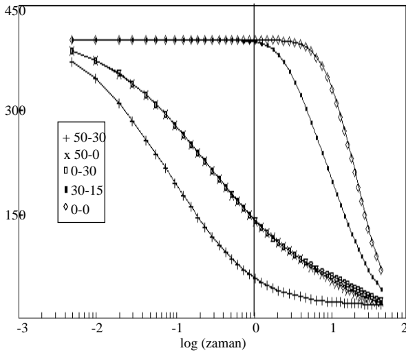
řekil 4. Kesit üzerindeki çeřitli noktalarda zamanla sıcaklık deęiřimi
