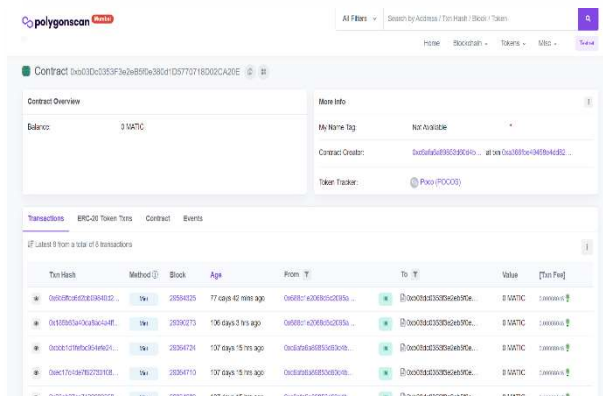
Figure 7.2. NFT Token Contract(ERC1155)
