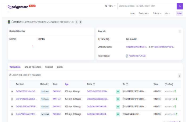
Figure 7.3. Token Contract(ERC 721)
